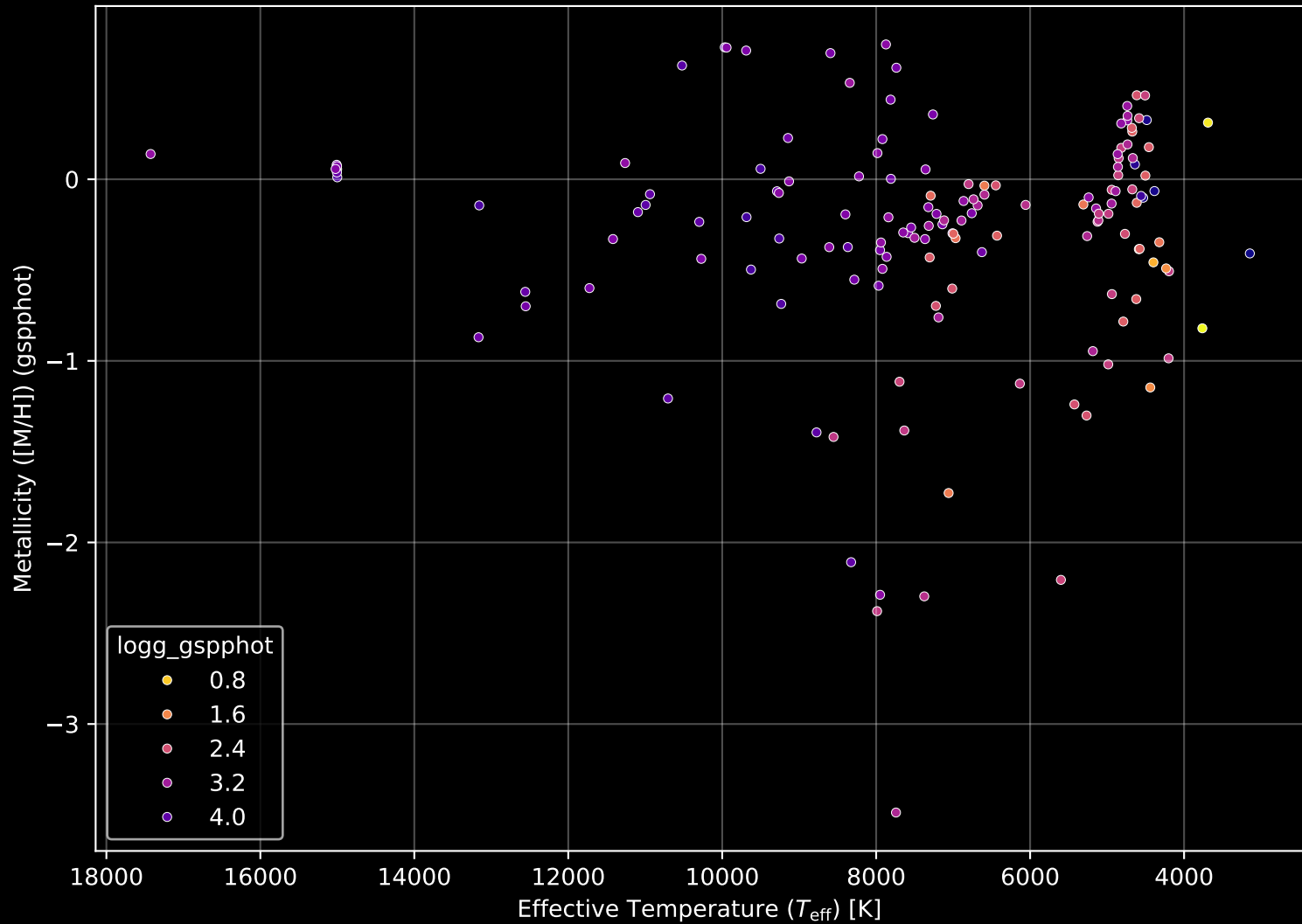
APOGEE DR17 Field: [143+00] Stellar Population Parameters (n= 152)
